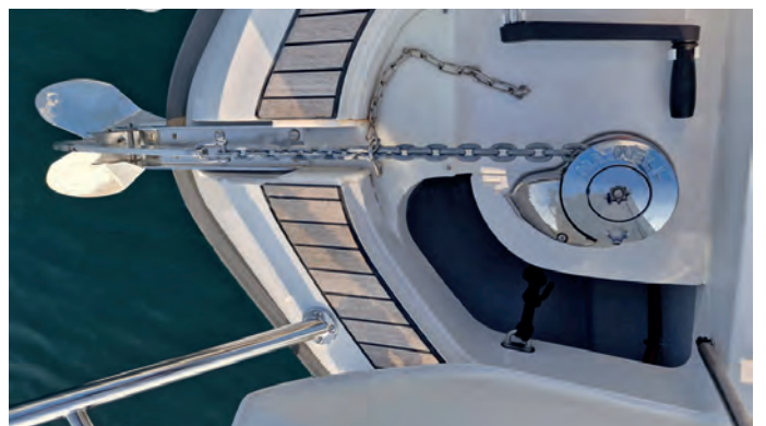
FM331113 스테인리스 체인 및 10kg 앵커 포함 선수 전동 윈들러스 (옵션 사양)
