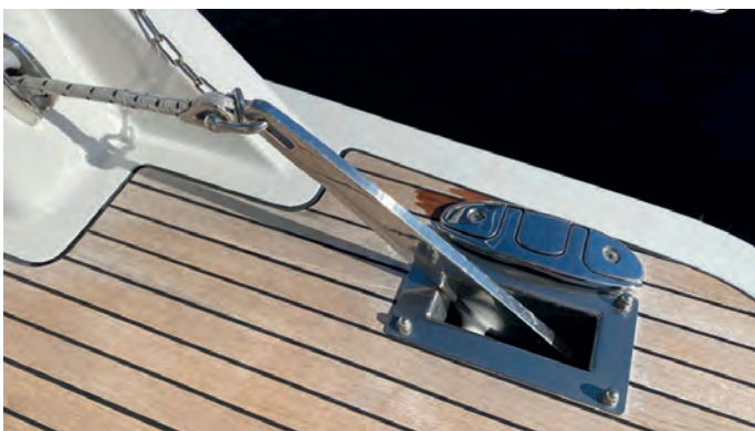
FM331494 후방 전동 윈들러스 Side-Power Maxi 1000W/12V 및 8kg 스테인리스 앵커 (옵션 사양)
